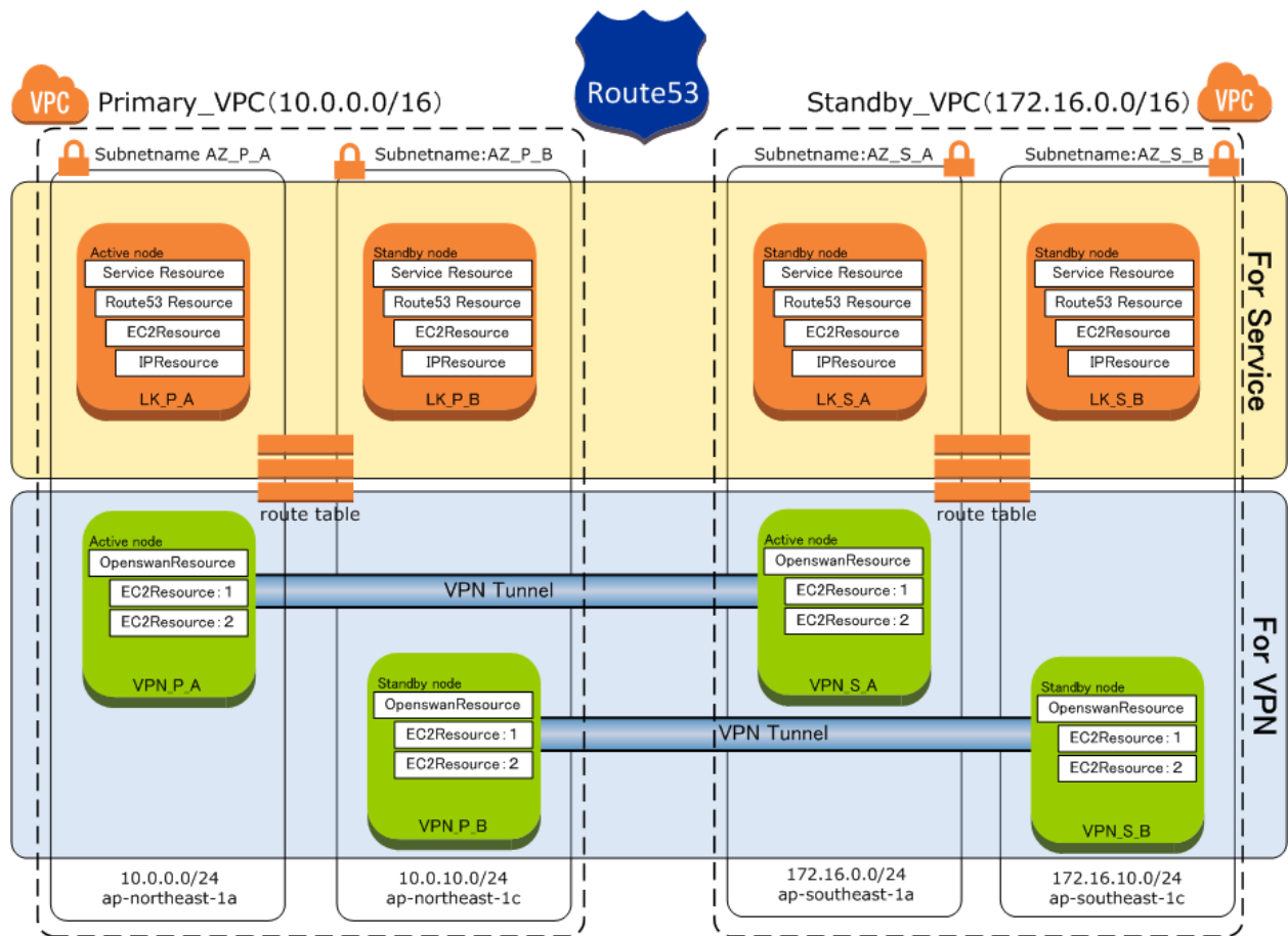
図 3 設定例の構成
