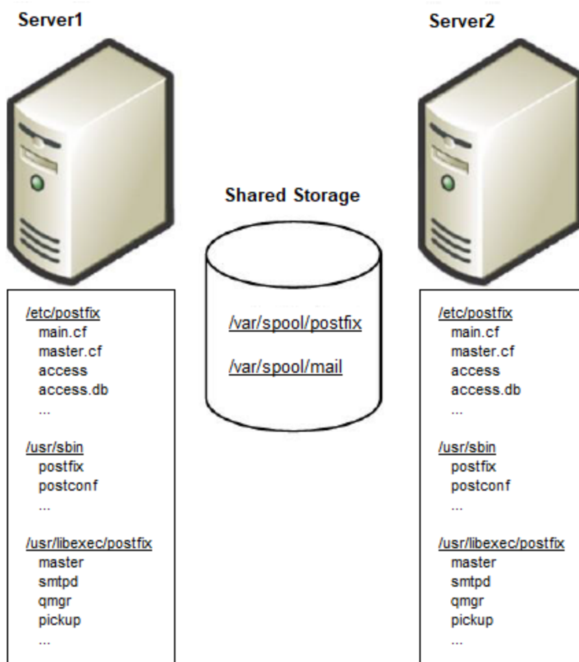
図1: 典型的なLifeKeeper アクティブ/スタンバイPostfix 環境 1
